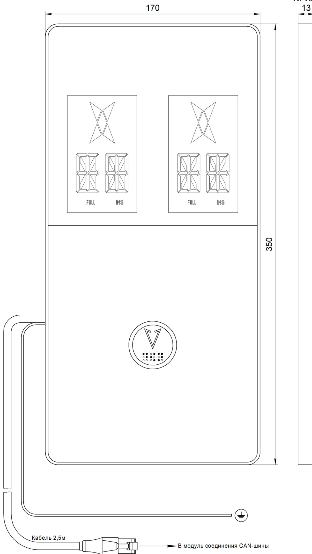
Рис.1 Внешний вид, габаритные и установочные размеры Вызывного поста МАЛАХИТ (жгут RJ45) НШЕК.468381.102
